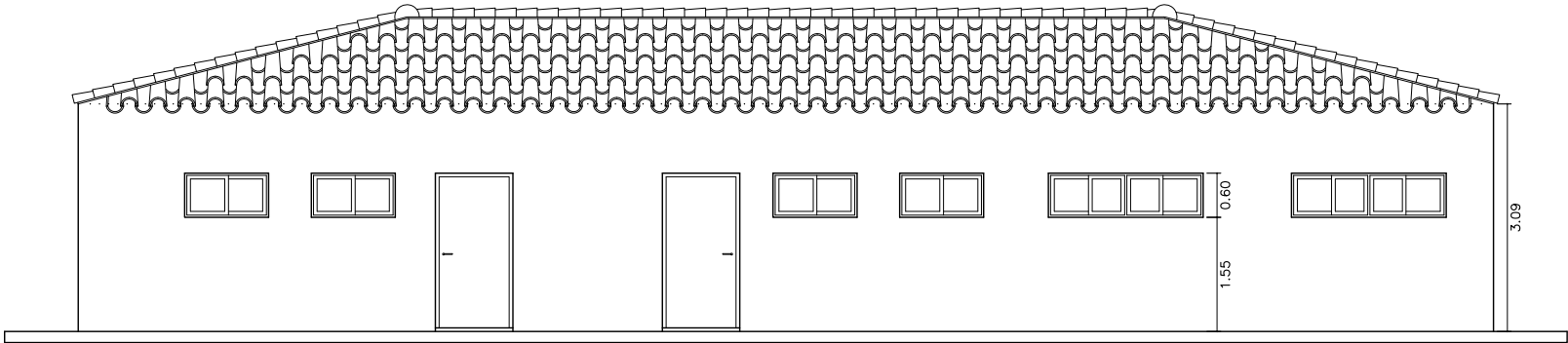
ALZADO SUR
