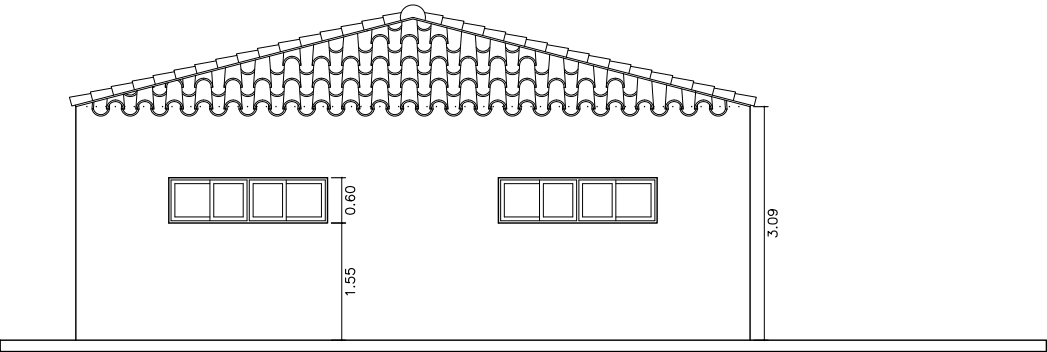
ALZADO ESTE
