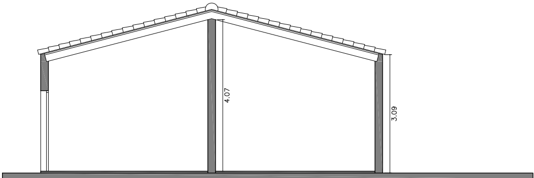
SECCIÓN TRANSVERSAL
