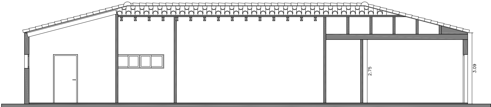
SECCIÓN LONGITUDINAL
