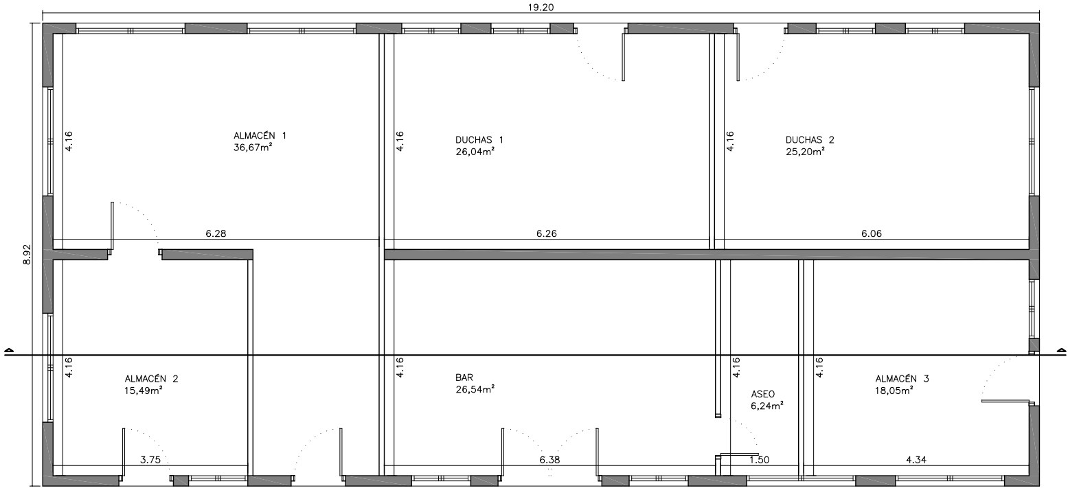
PLANTA BAJA
